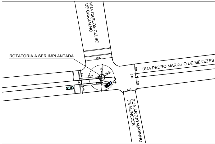
DETALHE ROTATÓRIA - IMPLANTAÇÃO ESCALA 1:250
