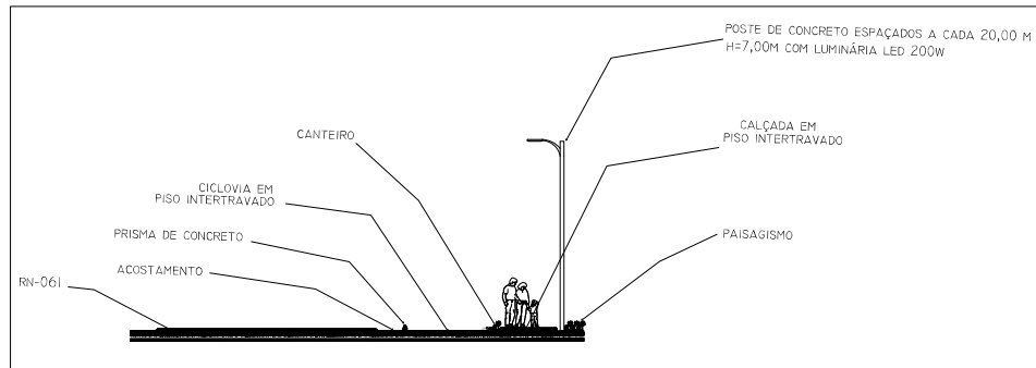
CORTE AA - URBANIZAÇÃO COM CICLOVIA E CALÇADAS ESCALA 1:100
